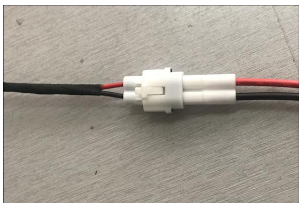
左右电机线红色线接红色线，黑色线接黑色线
