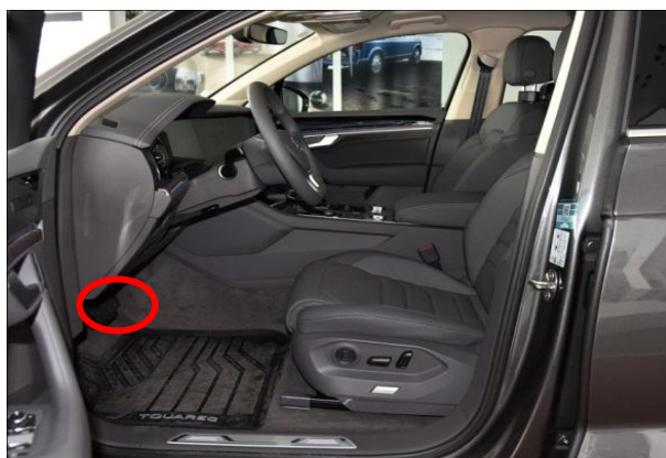
安装 ECU :在主驾找到 ECU 放置 ECU 的位置并用扎带固定；
